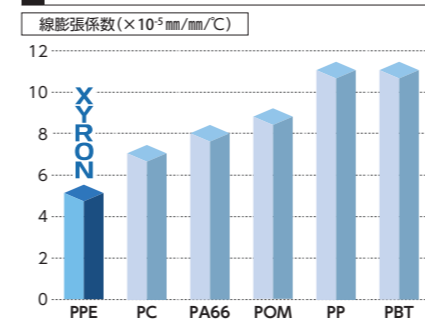
4 低線膨張係数 | 寸法安定性に優れます!
