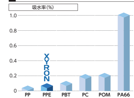
5 吸水率が低い | 耐水性に優れます!
