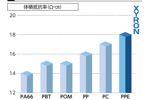
3 体積抵抗率が高い | 絶縁性に優れます!
