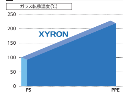
1 ガラス転移温度が高い | 耐熱性に優れます!
