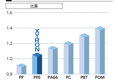
6 比重が小さい | 軽量化に貢献できます!
