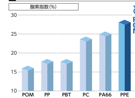
2 酸素指数が高い | 難燃性に優れます!
